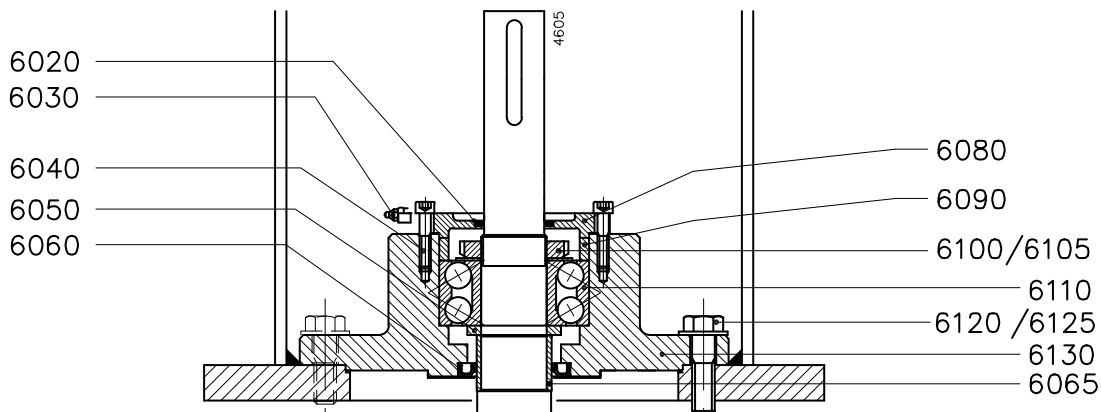
Figure 7: Roulement à billes.
